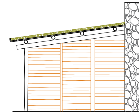
Alzado Anexo Cuadras
