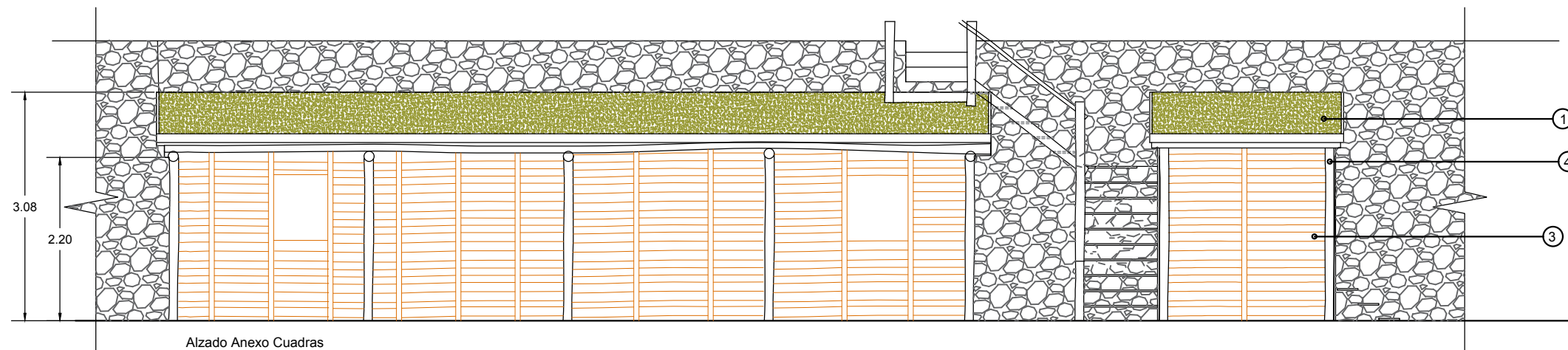
Alzado Anexo Cuadras
