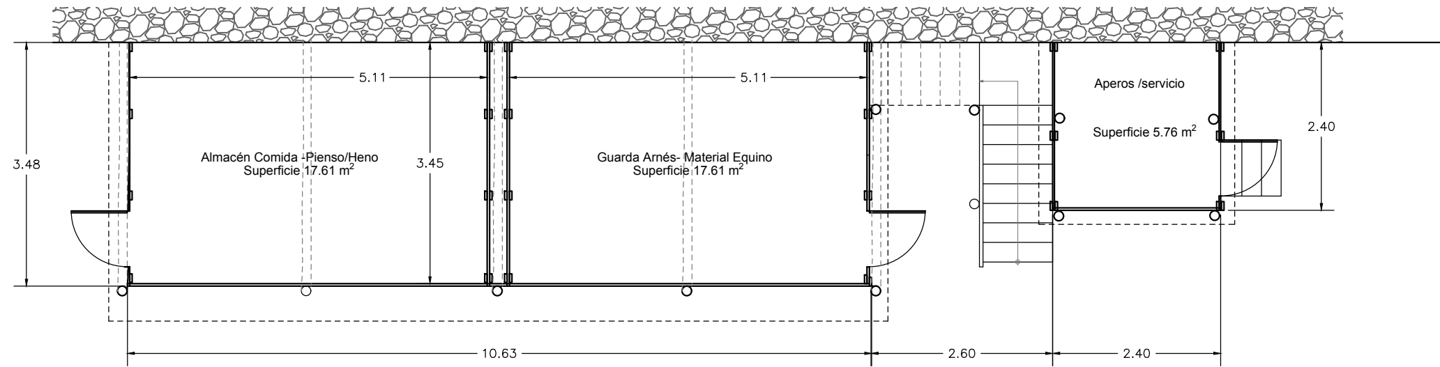
Planta Anexo Cuadras
